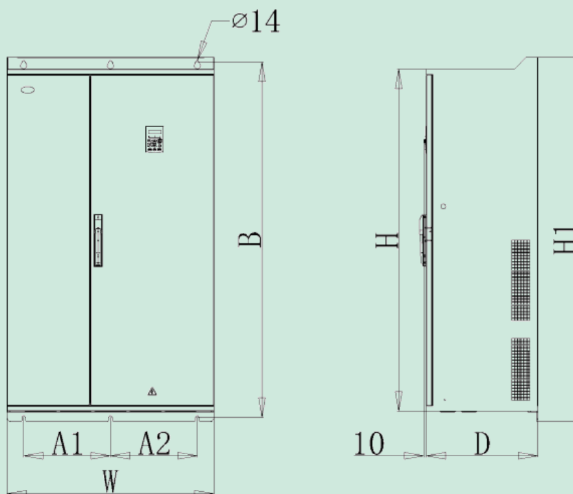
450kW~710kW 外形尺寸及安装尺寸示意图
