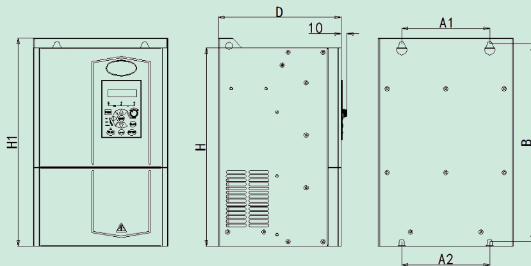
30 kW~132kW 外形尺寸及安装尺寸示意图
