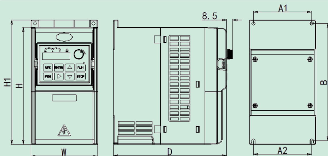
22kW 及以下功率外形及安装尺寸示意图
