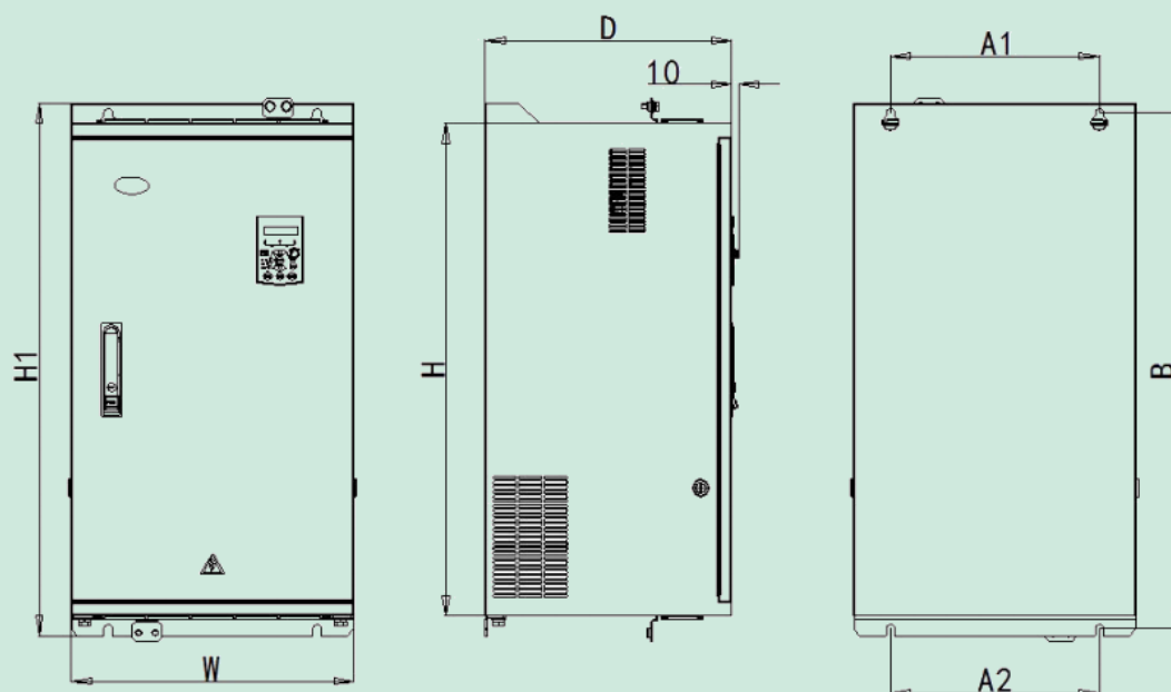
160kW~400kW 外形尺寸及安装尺寸示意图
